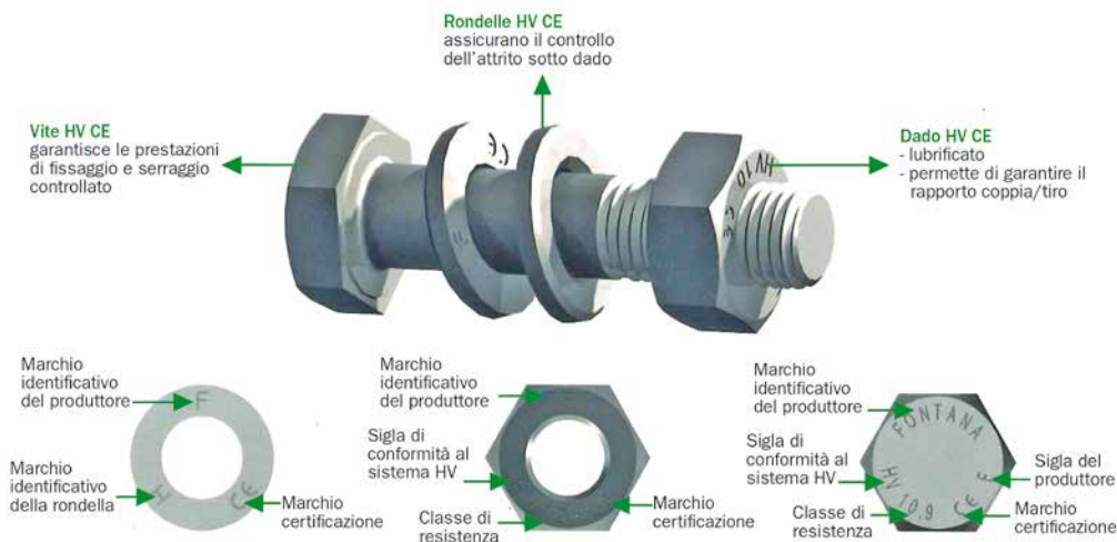
1. Gli assiemi Tecnosix ® HV da prearico vengono applicati per le costruzioni in acciaio
